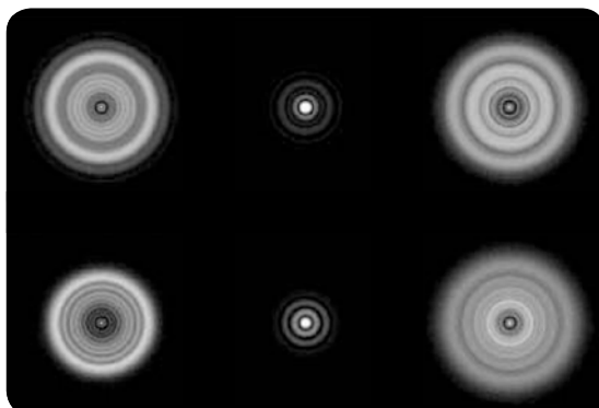
Sphärische Aberration
