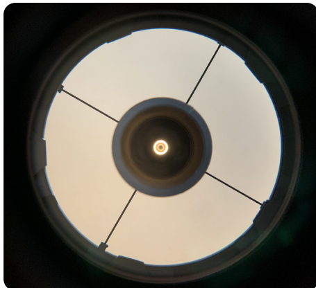
RC-Teleskop mit korrekt eingestelltem Sekundärspiegel, aber dejustiertem Hauptspiegel; TSCOLLIT auf Fangspiegelspinne scharfgestellt.
