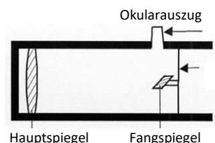
Hauptspiegel Fangspiegel
