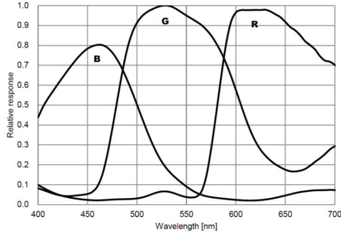
Abbildung 2 IMX294 Spektrale Empfindlichkeitscharakteristik
