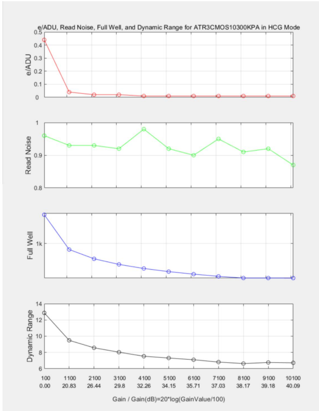
Abbildung 6 e-/ADU, Lese-Rauschen, Full Well und Dynamikbereich für ATR294C
