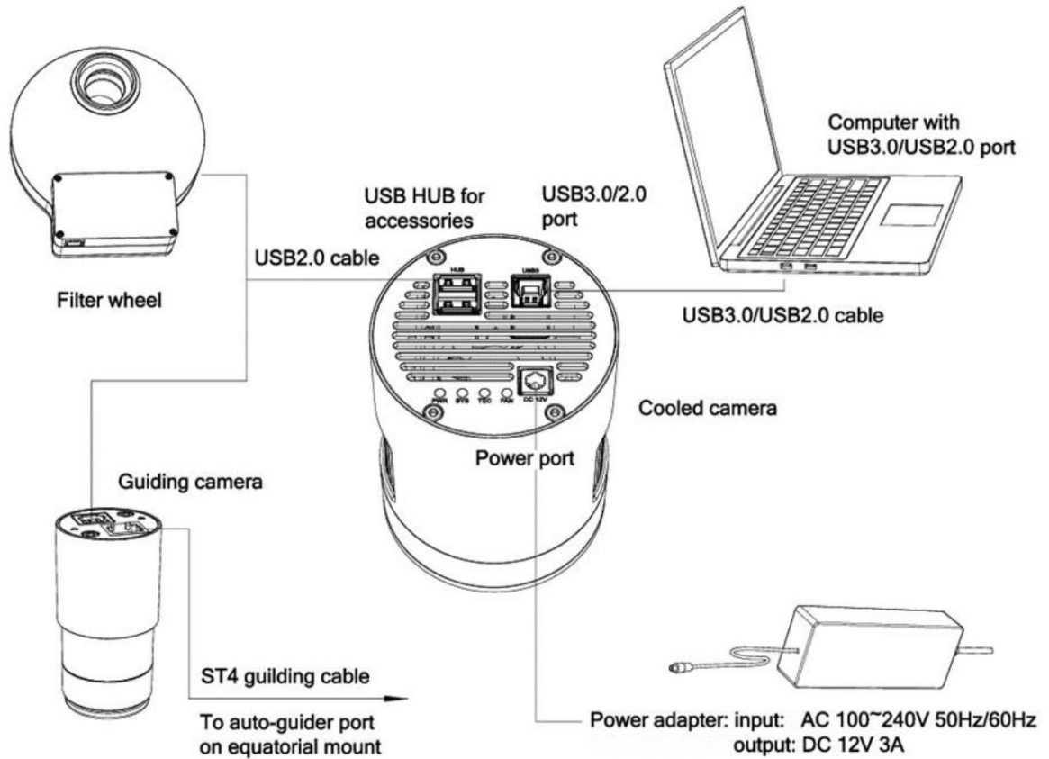
Abbildung 12 Elektrischer Anschluss der Kamera
