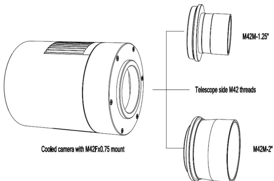
Abbildung 10 Die Verbindung von ATR-Kamera und Adapter
