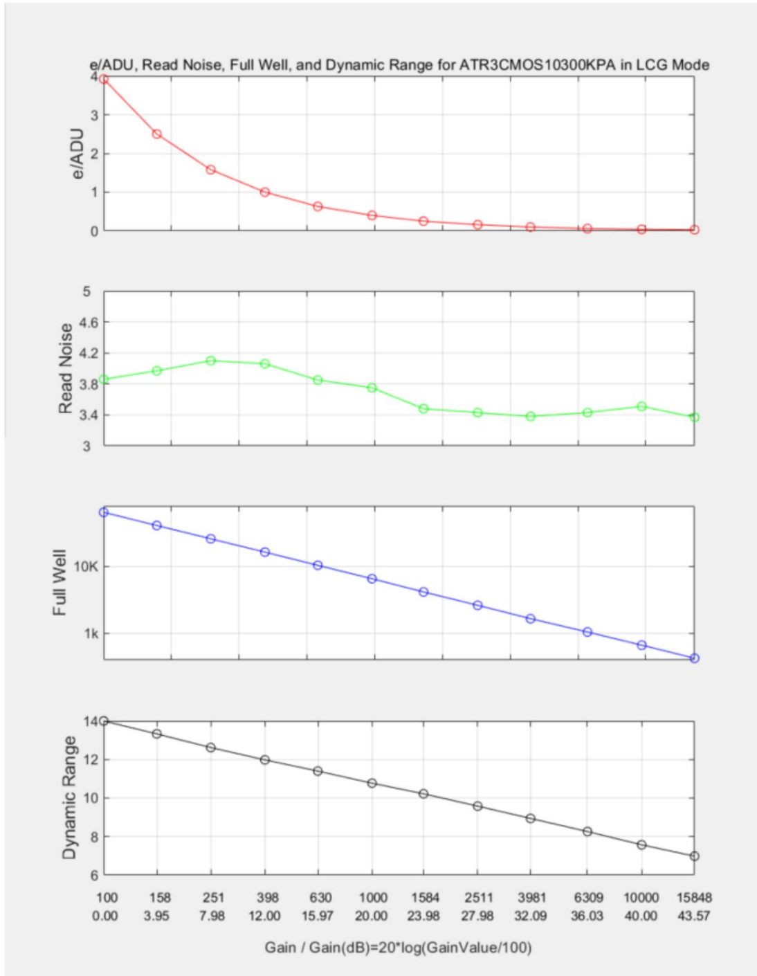
Abbildung 5 e-/ADU, Lese-Rauschen, Full Well und Dynamikbereich für ATR294C
