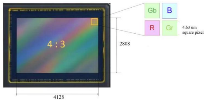
Abbildung 1 IMX294-Sensor und seine Pixelstruktur
