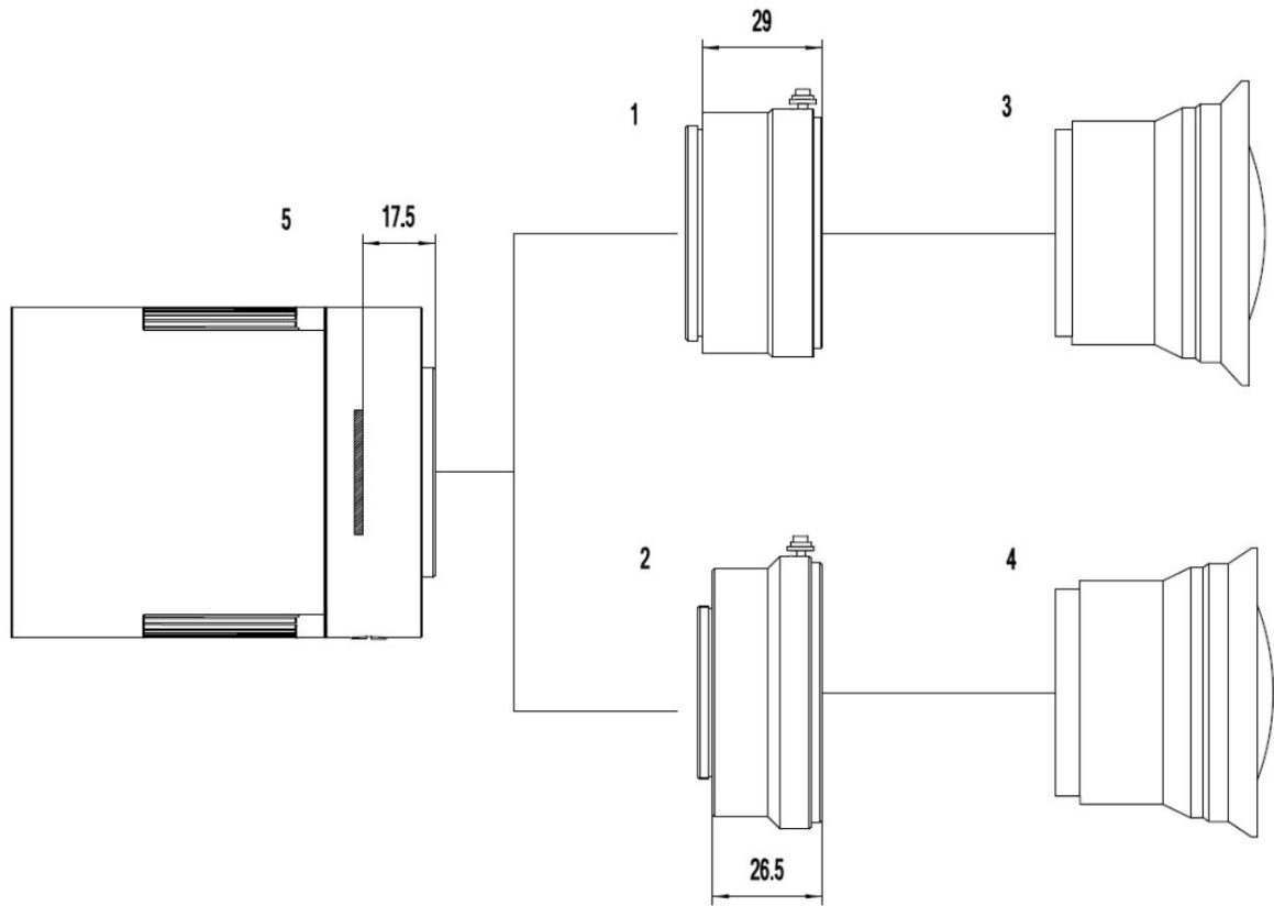
Abbildung 13 Nikon F/Canon EF-Objektiv mit ATR-Kamera
