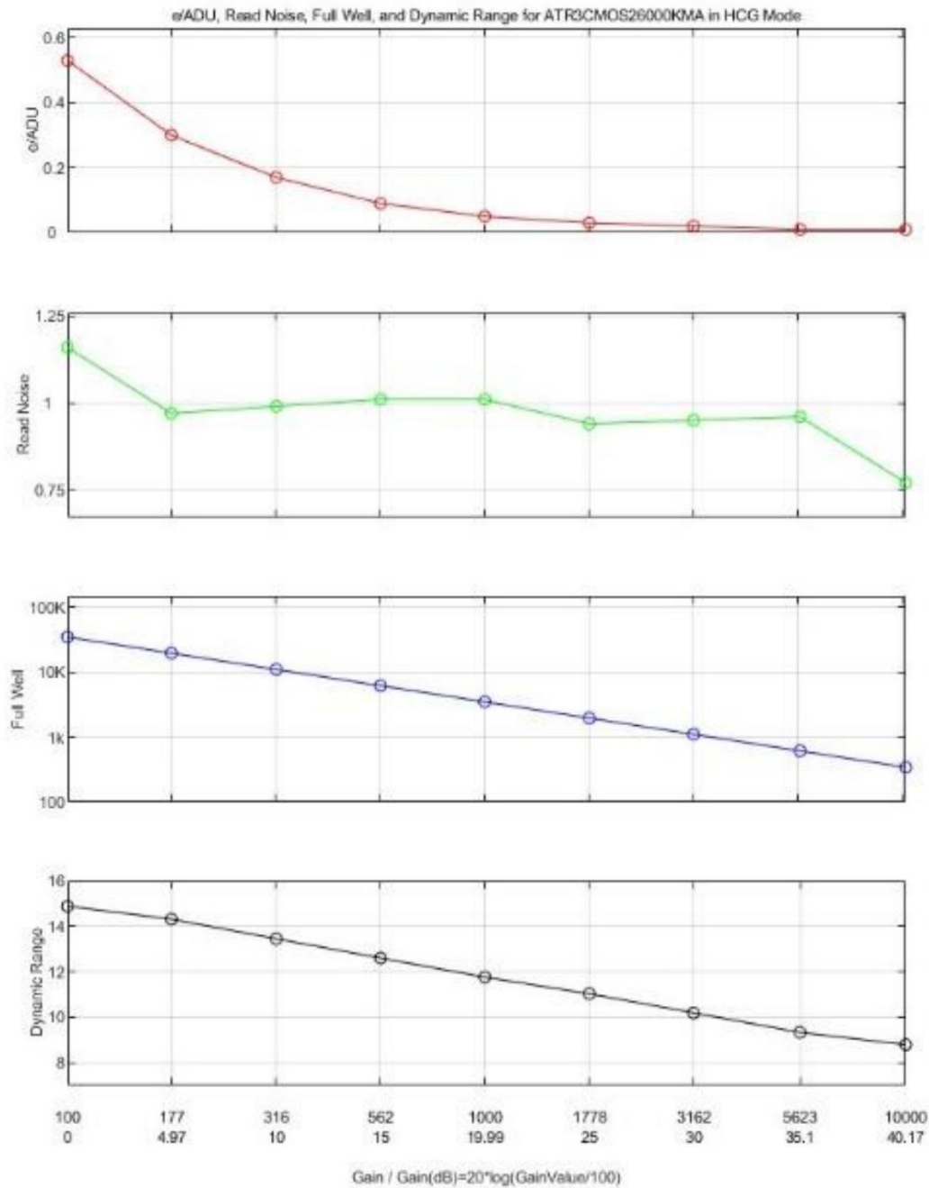
Abbildung 6.1 e/ADU, Lese-Rauschen, Full Well und Dynamikbereich für ATR2600M
