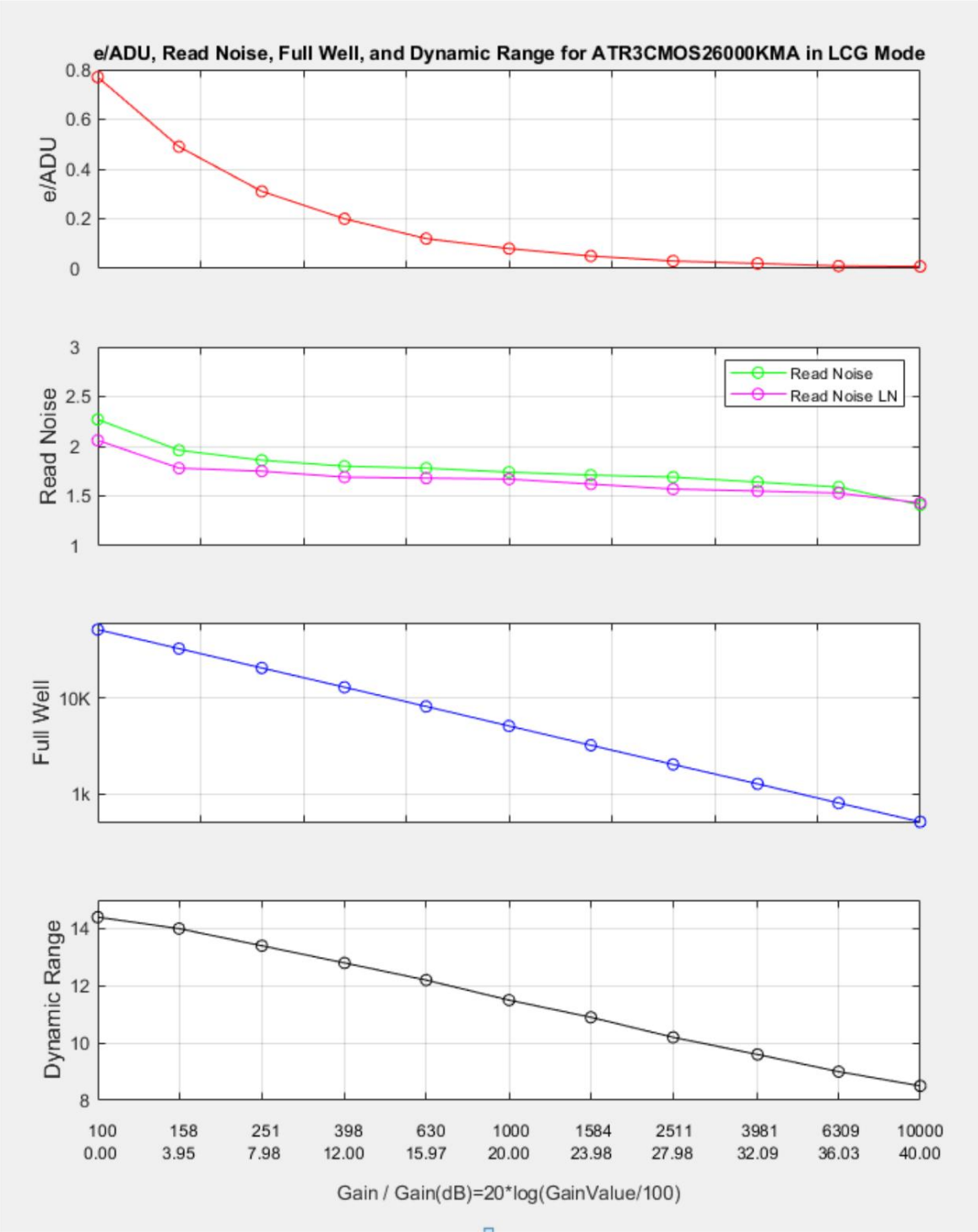
Abbildung 7 e/ADU, Lese-Rauschen, Full Well und Dynamikbereich für ATR2600M
