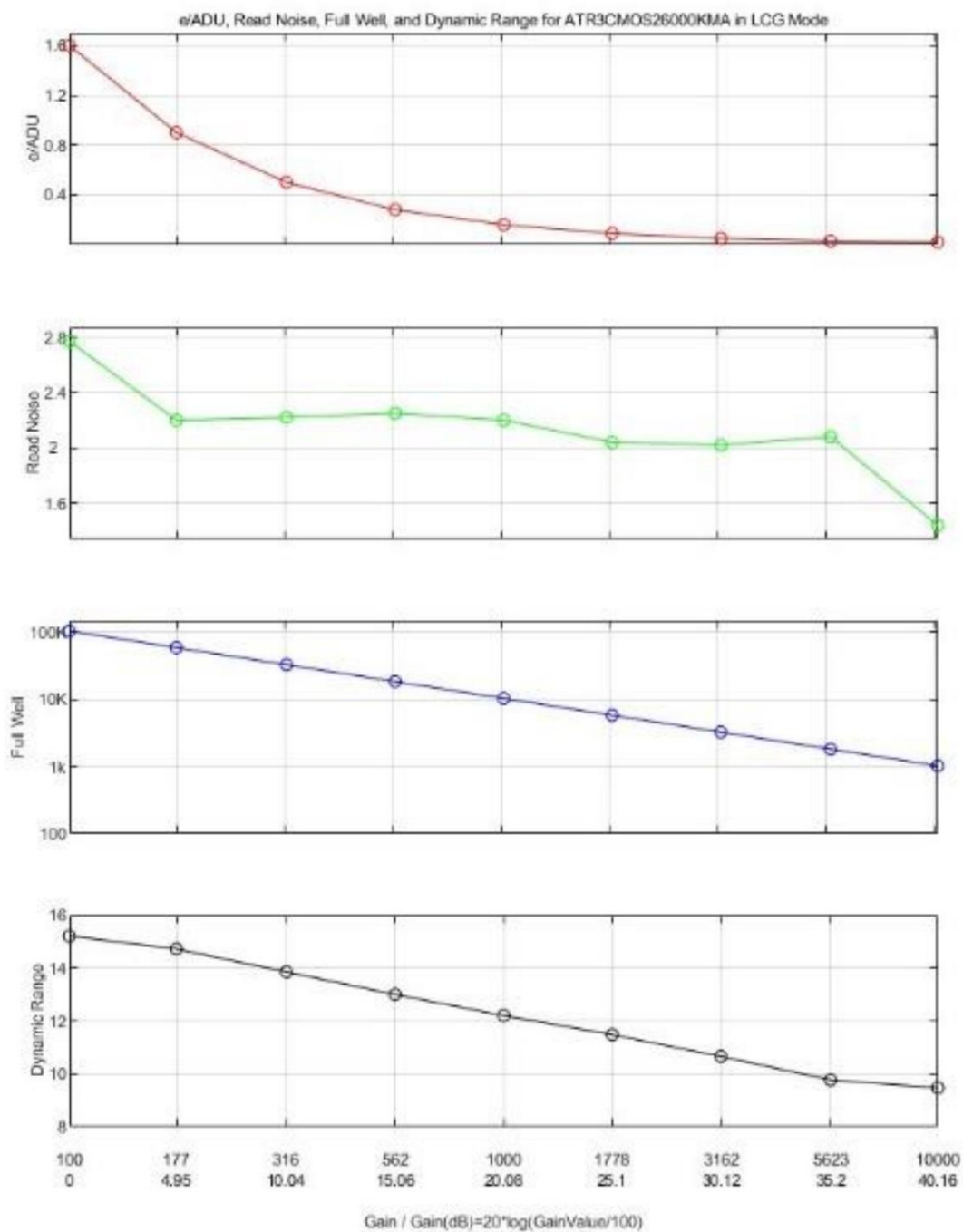
Abbildung 8.1 e/ADU, Lese-Rauschen, Full Well und Dynamikbereich für ATR2600M
