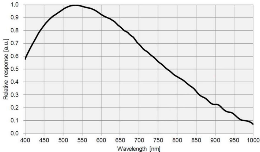
Abbildung 2 IMX571 Spektrale Empfindlichkeitscharakteristik
