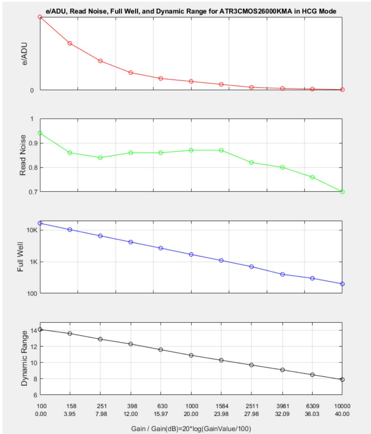
Abbildung 5 e/ADU, Lese-Rauschen, Full Well und Dynamikbereich für ATR2600M
