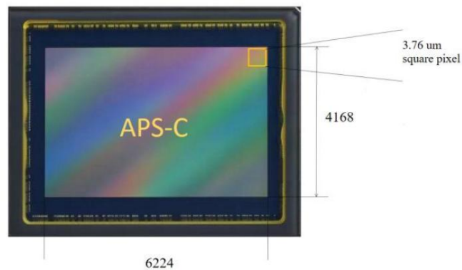
Abbildung 1 IMX571-Sensor und seine Pixelstruktur
