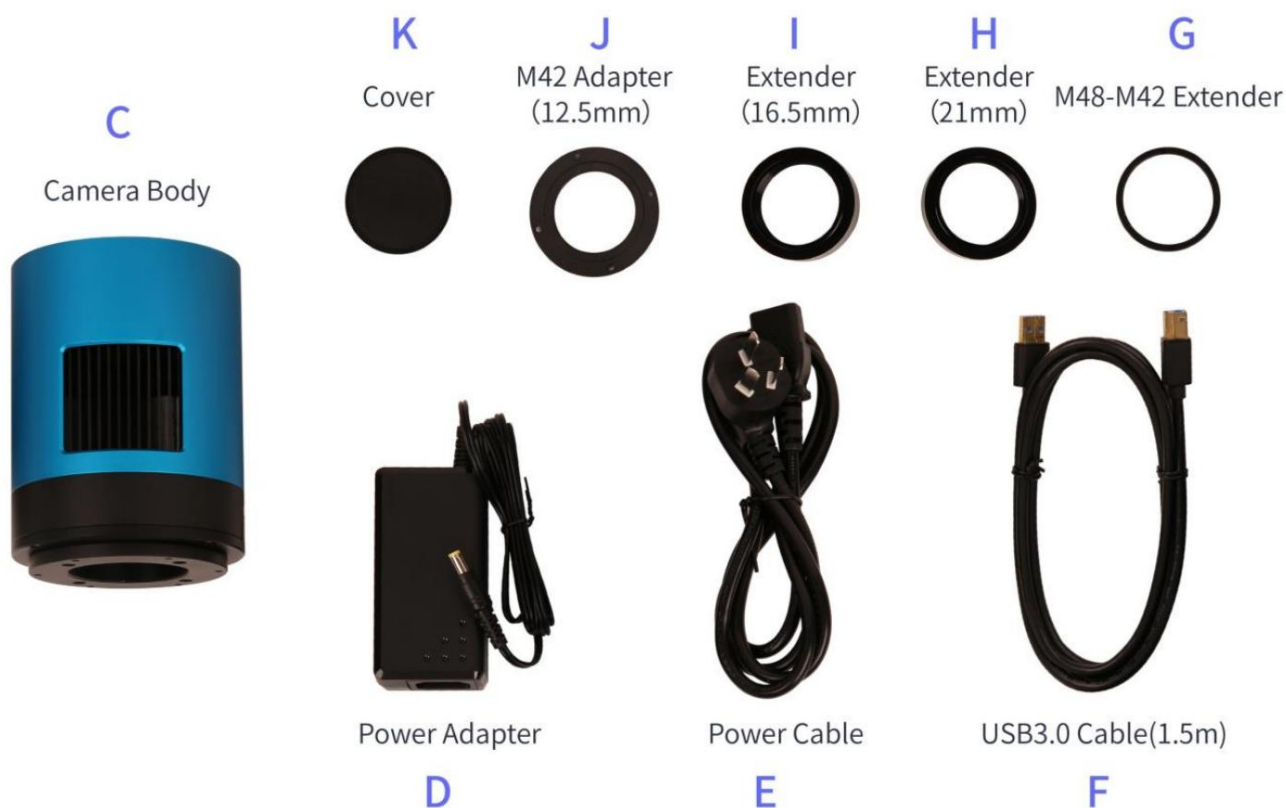
Abbildung 9 Verpackungsinformationen für ATR2600M
