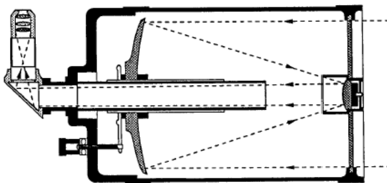
Figura 3-1 Esquema del diseño óptico del sistema Schmidt-Cassegrain
