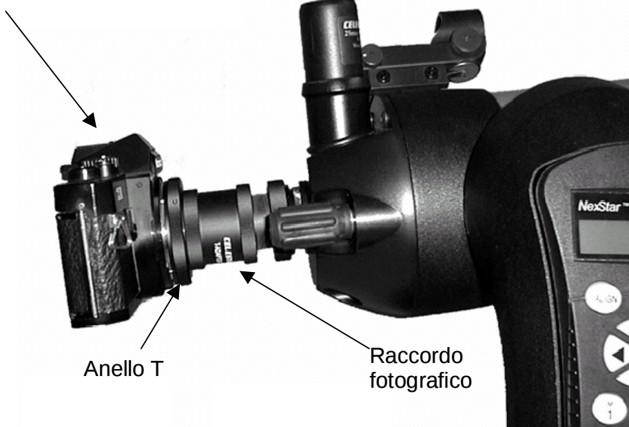
Fotocamera Reflex
