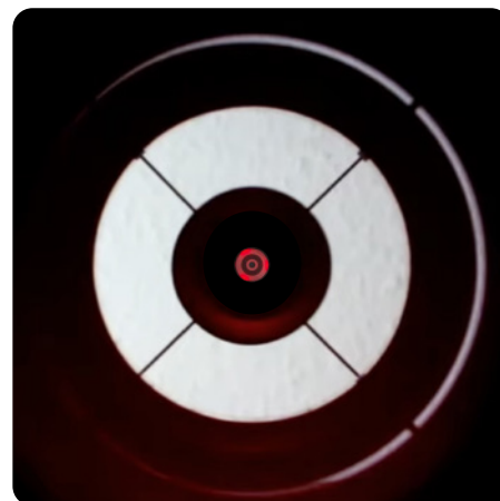
RC-Teleskop mit korrekt eingestelltem Sekundärspiegel, aber falsch ausgerichtetem Primärspiegel.
